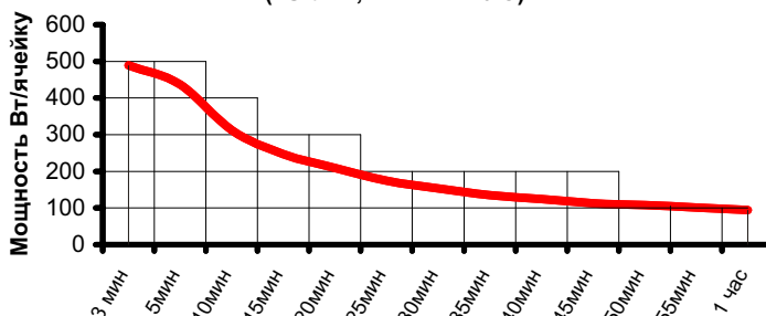
Разряд постоянной мощностью ( U_{\text{кон}}=1,7 \text{ В} T=20^\circ\text{C} )
