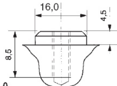
Винт М6
