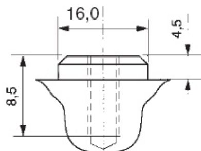
Винт М5
