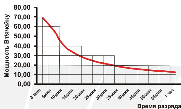
Разряд постоянной мощностью ( U_{кон}=1,7 В T=20^{\circ}C )
