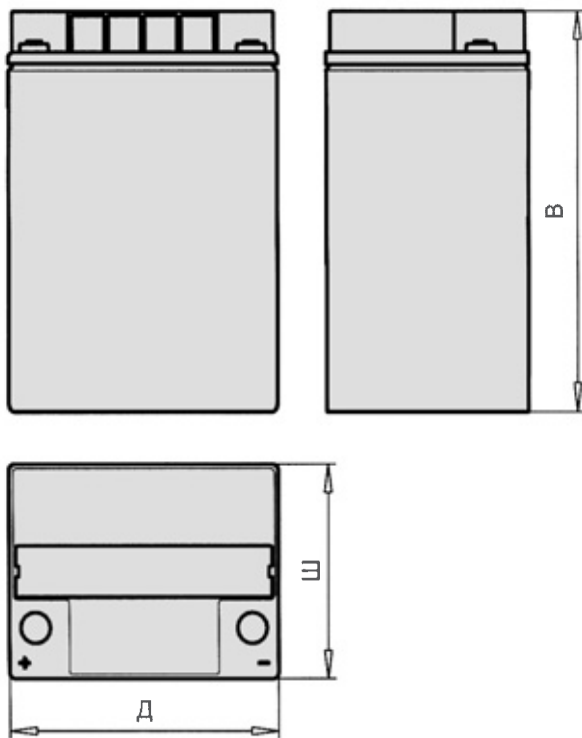
12 V 1 OPzV 50 - 12 V 3 OPzV 150
